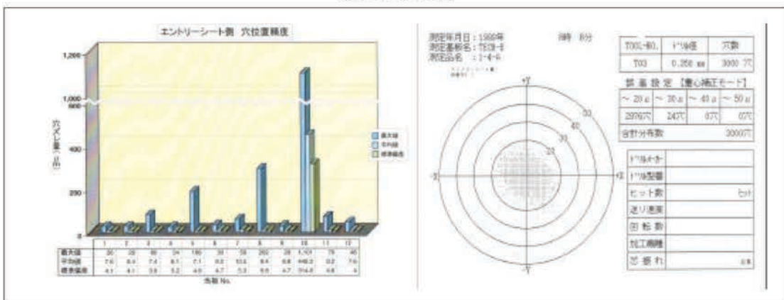
穴位置精度測定結果
