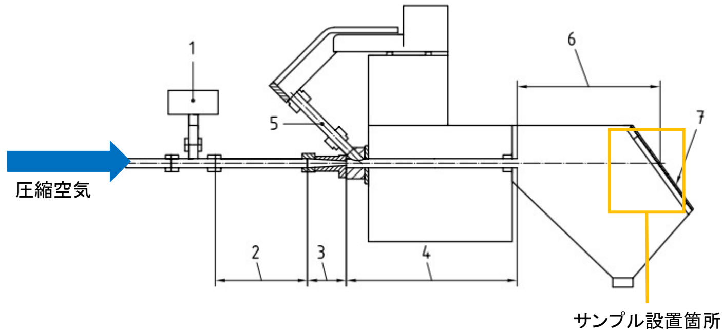
図. 試験装置拡大図
